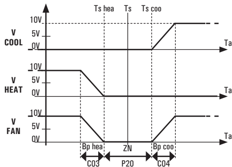
Abb. 14: Das Schema zeigt die Ventilsteuerung in einem 4-Leitersystem, mit Neutralzone. Im Diagramm wird angenommen, dass die Ventile proportional mit 0...10 V angesteuert und kein weiterer Einflüsse berücksichtigt werden. Wird ein 2-Leitersystem verwendet, wird das zugehörige Ventil in gleicher Weise angesteuert. Die Temperatur T_s ( Solltemperatur ) würde mit T_{s\ hea} zusammenfallen, bei aktivem Heizbetrieb und T_{s\ coo} im Kühlbetrieb.
